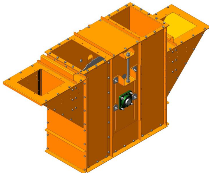
Рис. 2 Головка нижняя
