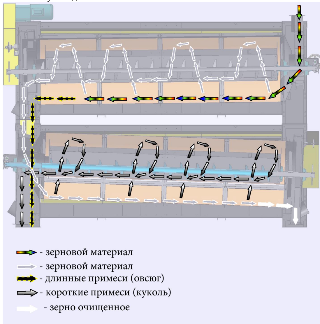
Рис. 2 Технологическая схема
