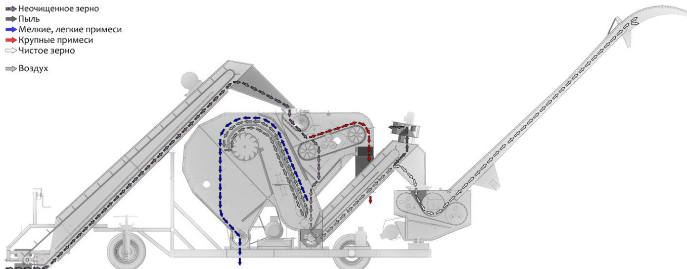
Рис. 2 Технологическая схема
