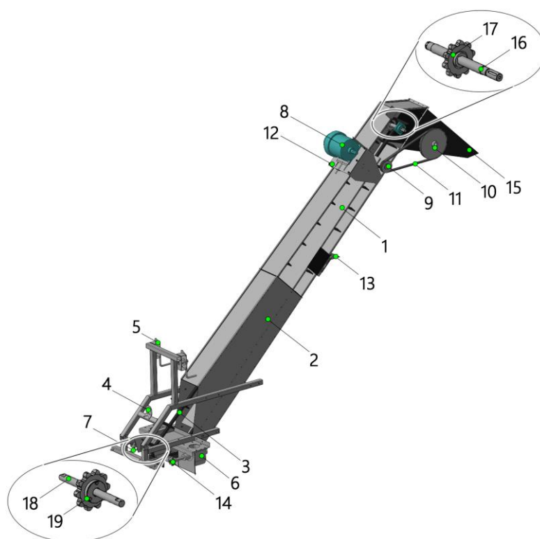
Рис. 6 Транспортер загрузочный
