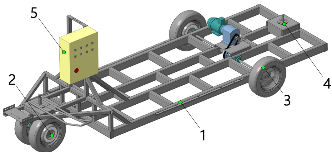
Рис. 4 Рама
