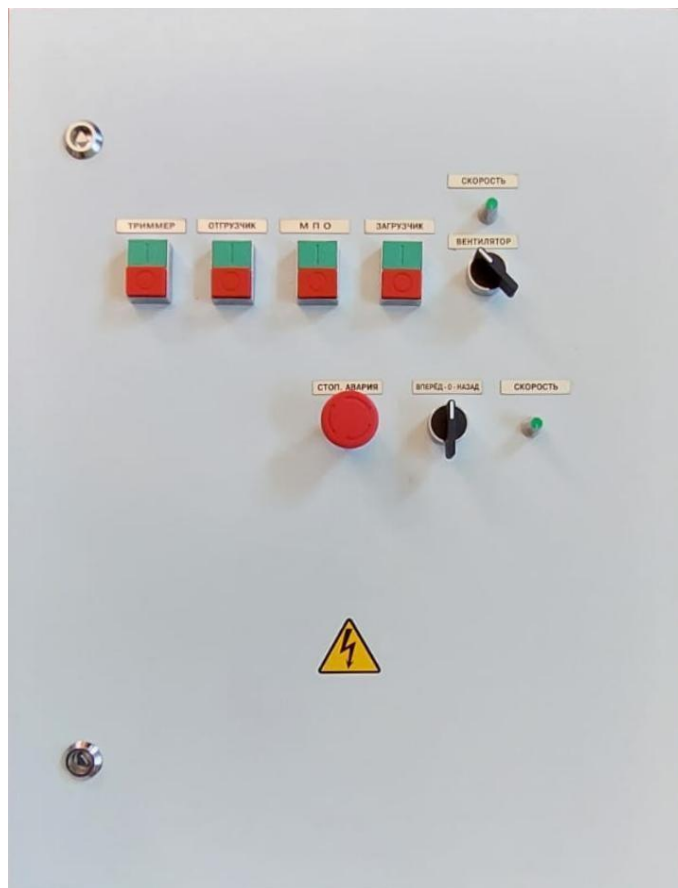
Рис. 15 Щит управления
