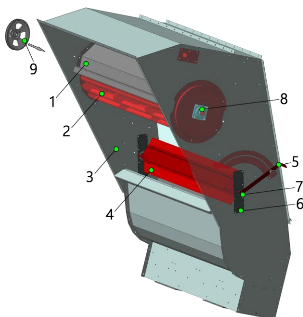
Рис. 9 Воздушная камера
