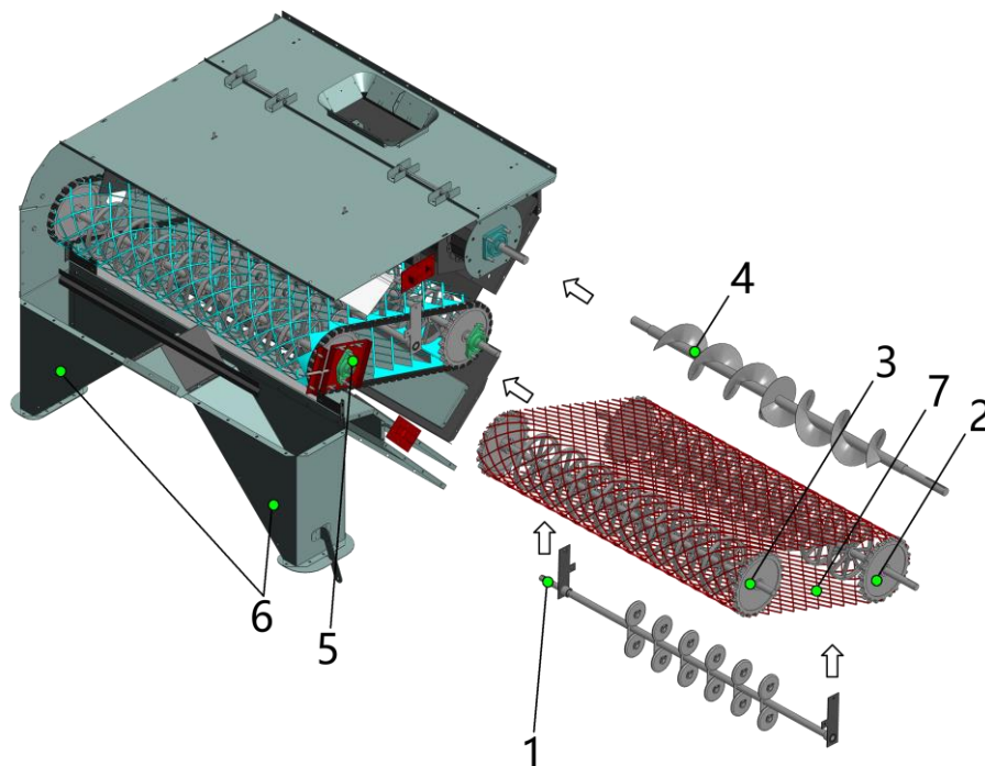
Рис. 8 Сетчатый транспортёр
