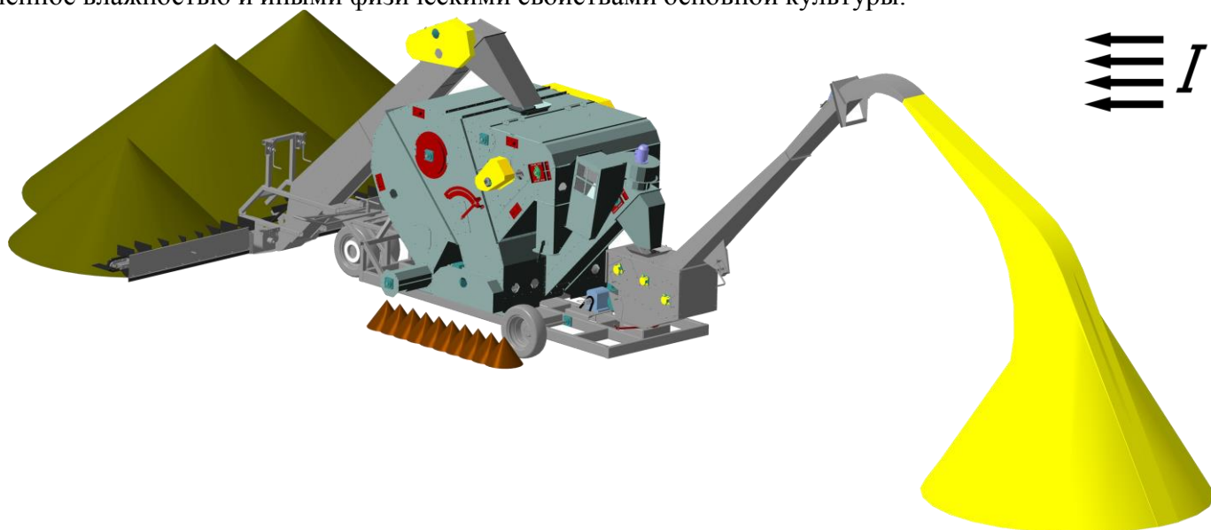
Рис. 3 Схема организации работ на току
