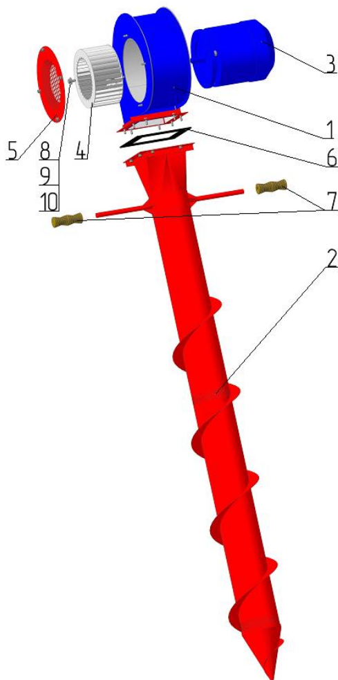
Рис.2 – Аэратор зерна АЗР-1.
