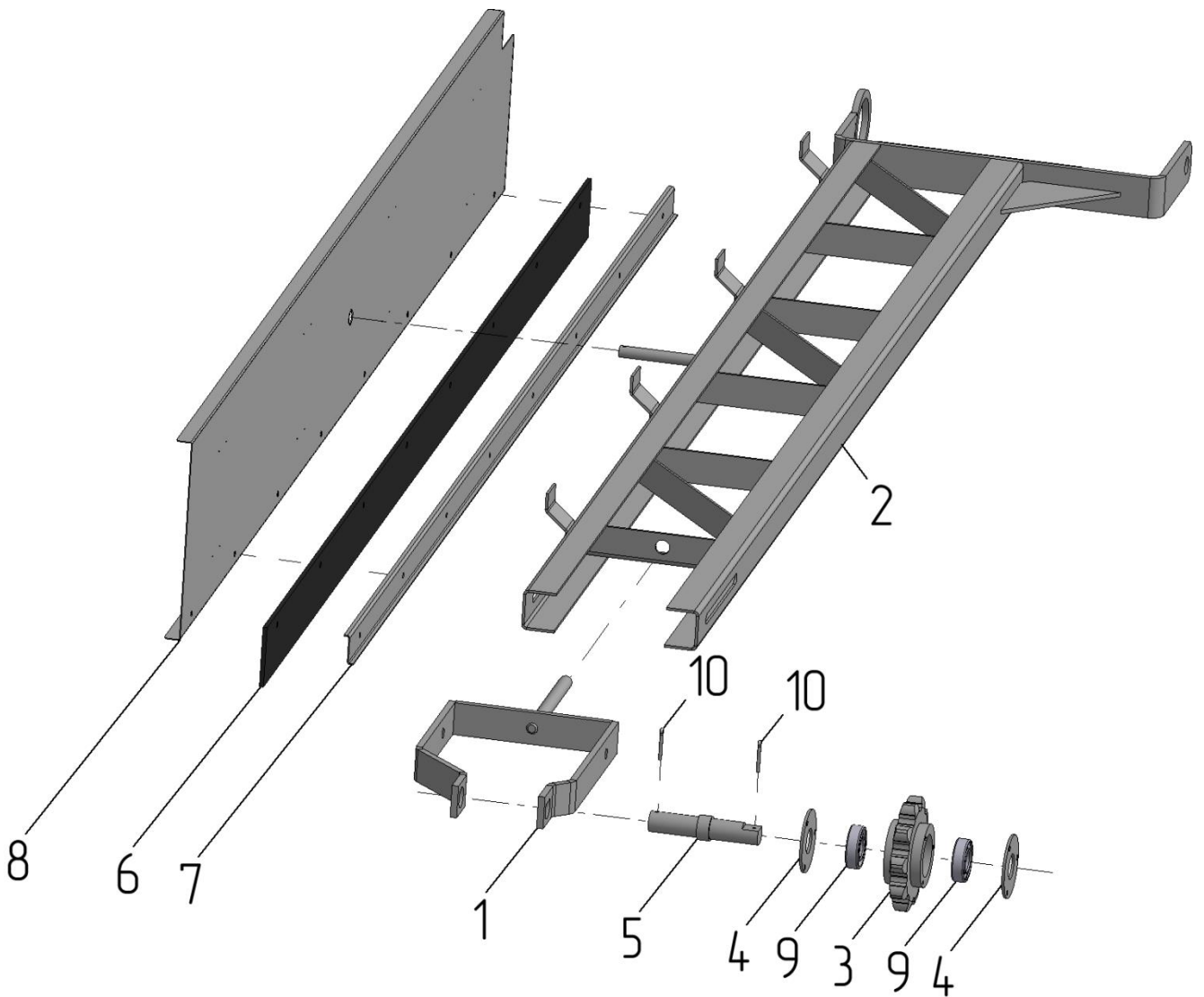
Рис. 9 - Питатель левый А 100-05.00
