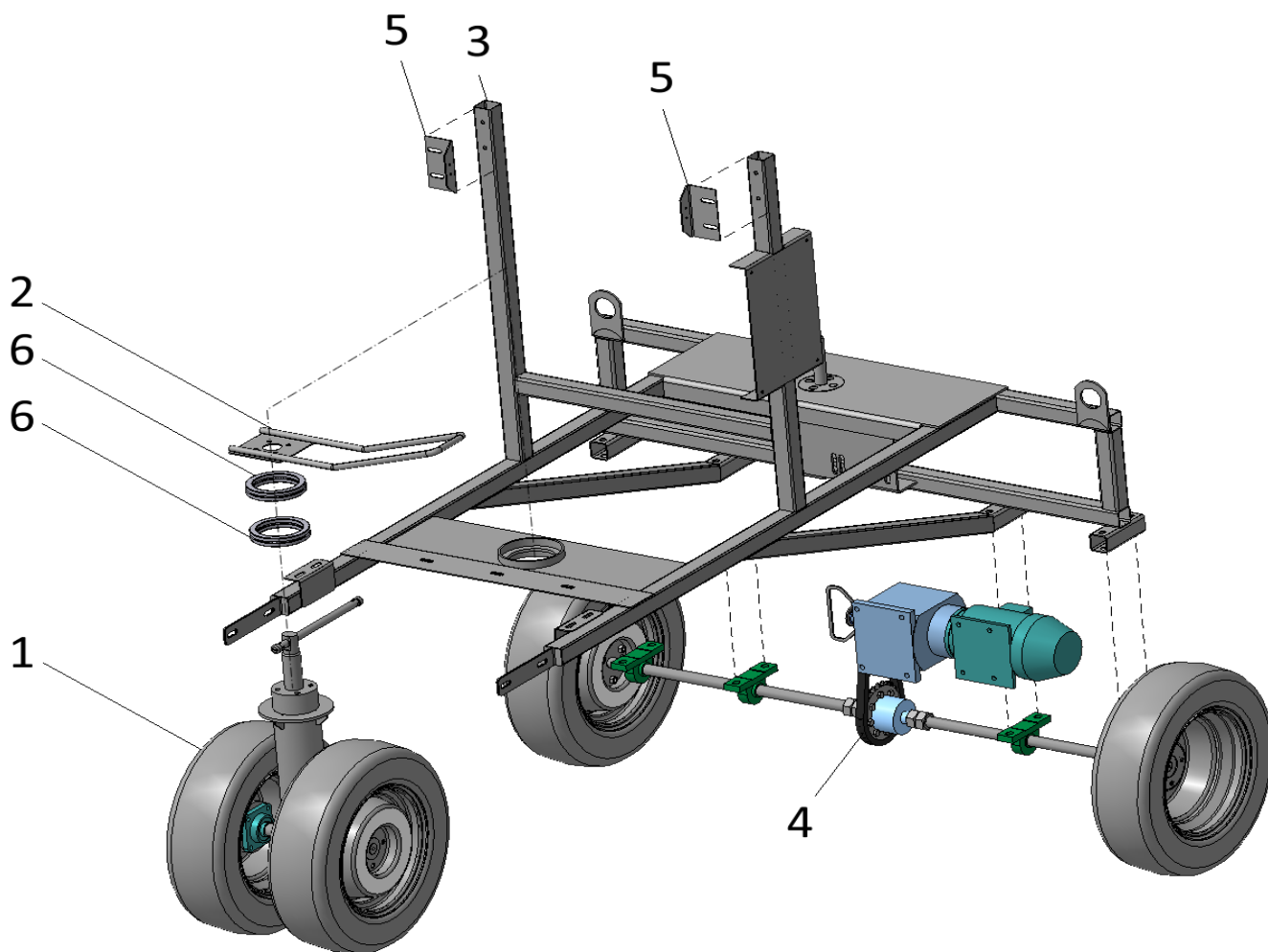
Рис. 4 - Рама опорная А 150-02.00
