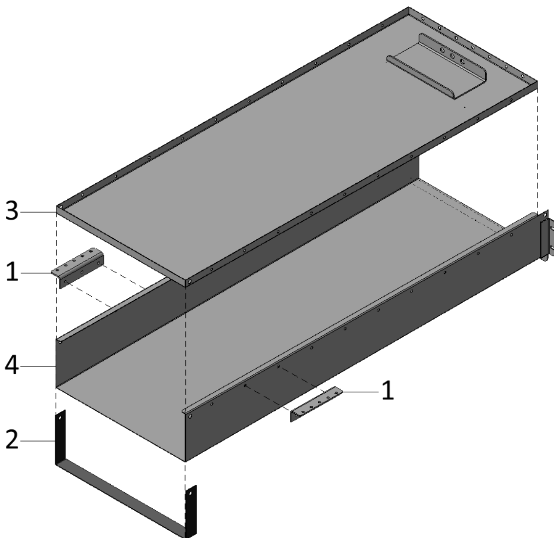
Рис. 15 - Лоток А 150-07.04.02
