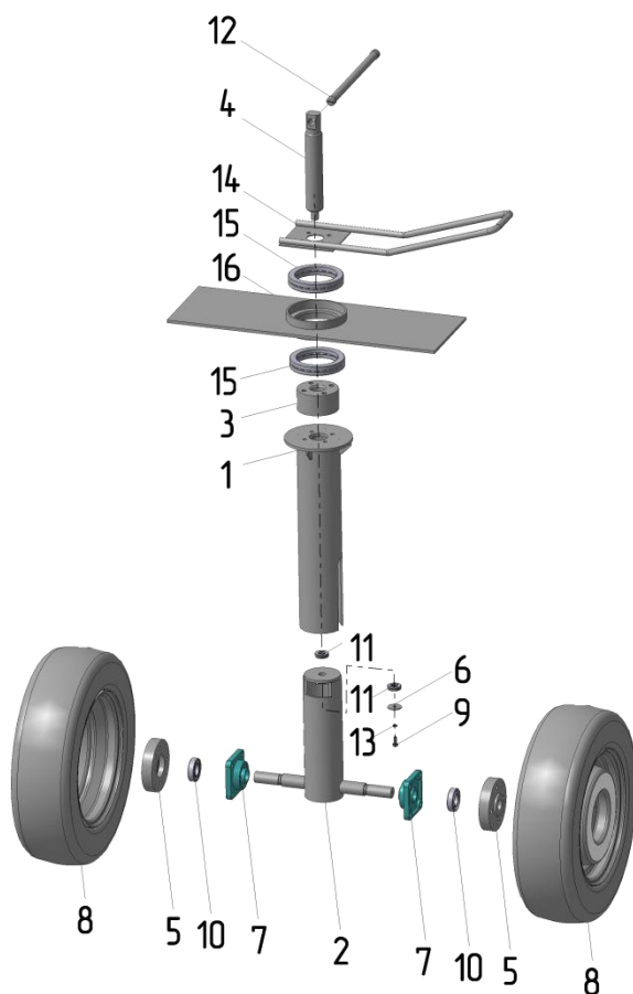
Рис. 5 - Колесо А 100-02.01.00
