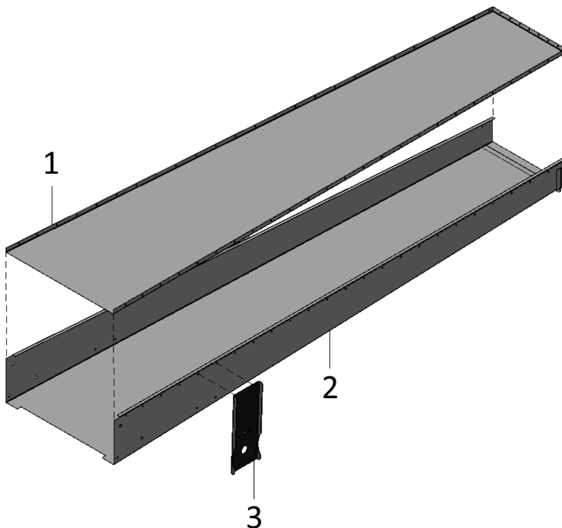
Рис. 14 - Лоток А 150-07.04.01
