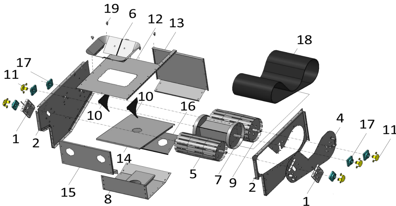
Рис. 12 - Триммер А 100-07.03.00
